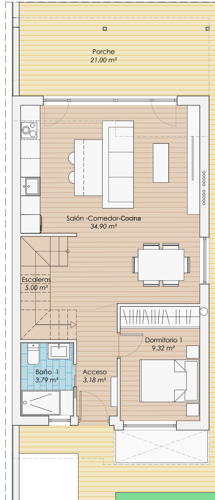
PLANTA BAJA Sup. útil 56,19 m 2 Sup. construida 65,87 m 2
