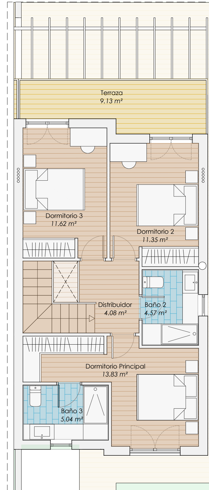
PLANTA PRIMERA Sup. útil 59,62 m 2 Sup. construida 66,17 m 2
