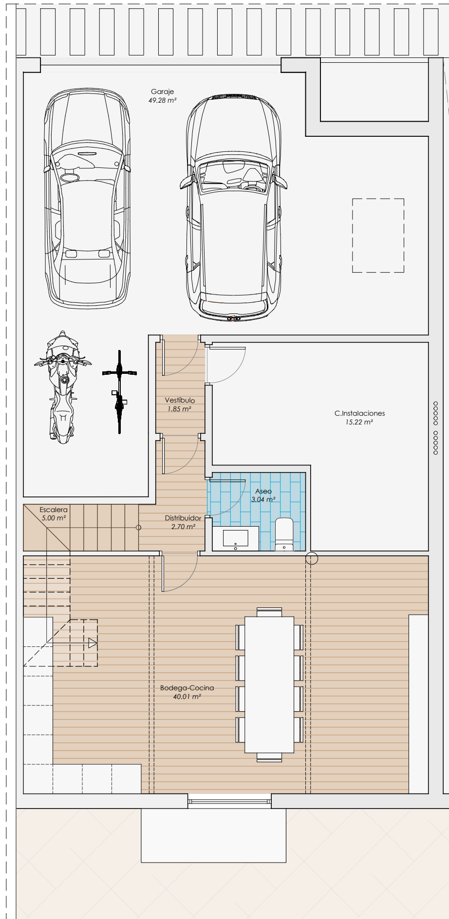
PLANTA SÓTANO Sup. útil 117,10 m 2 Sup. construida 129,87 m 2
